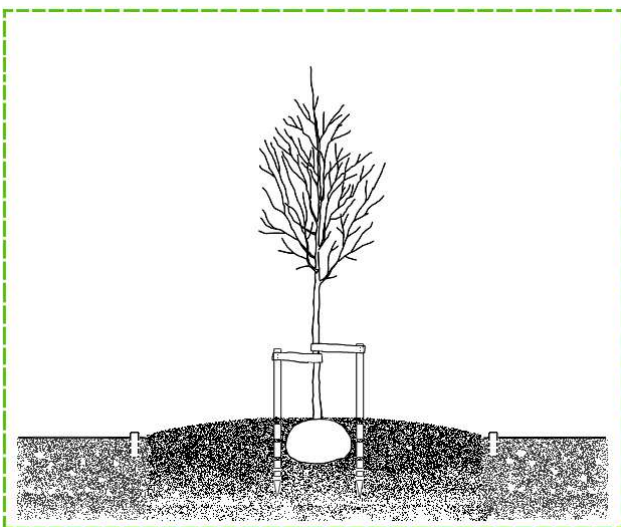
Figur 12. Upphöjd växtbädd när växtbäddens botten är mindre stabil. Ca 15 % sättning av en ditforslad eller djuplucrad jord är ett vanligt riktvärde.
